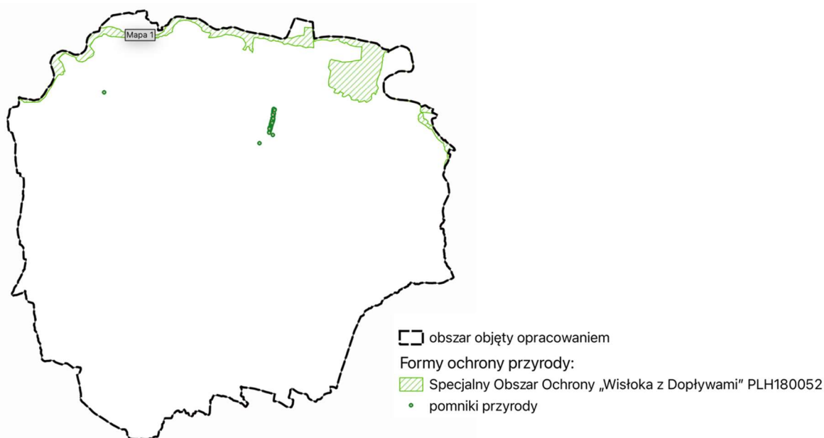
Rysunek 9 Formy ochrony przyrody w obszarze opracowania
