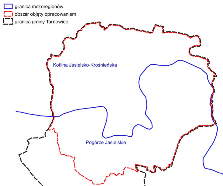
Rysunek 2 Położenie obszaru objętego planem względem jednostek fizycznogeograficznych wg Kondrackiego
