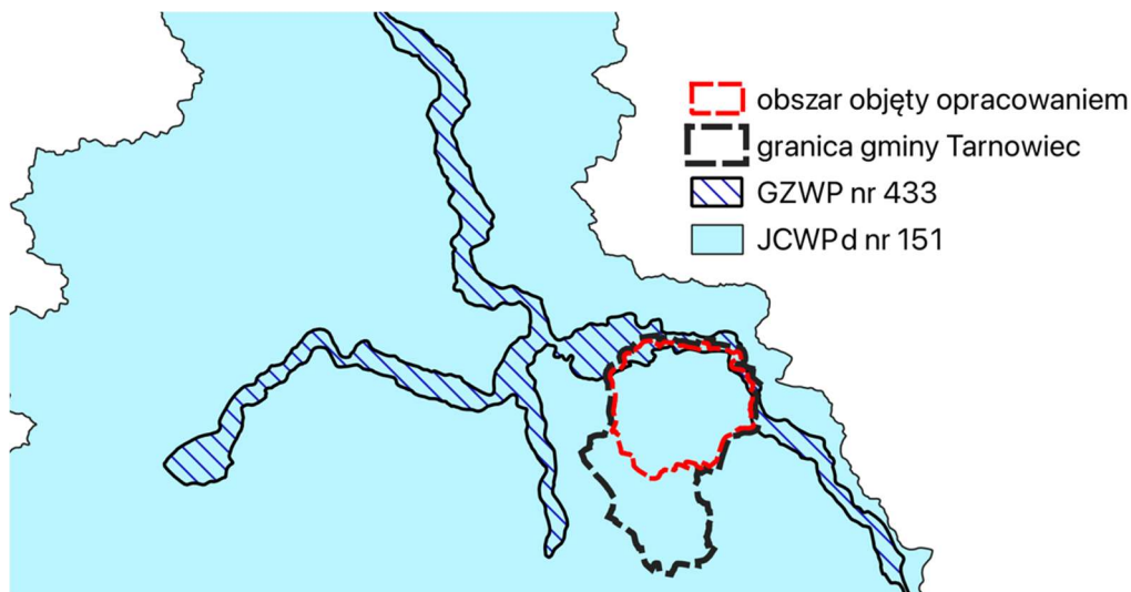
Rysunek 5 Położenie obszaru objętego planem względem Jednolitej Części Wód Podziemnych Nr 151 oraz GZWP nr 433
