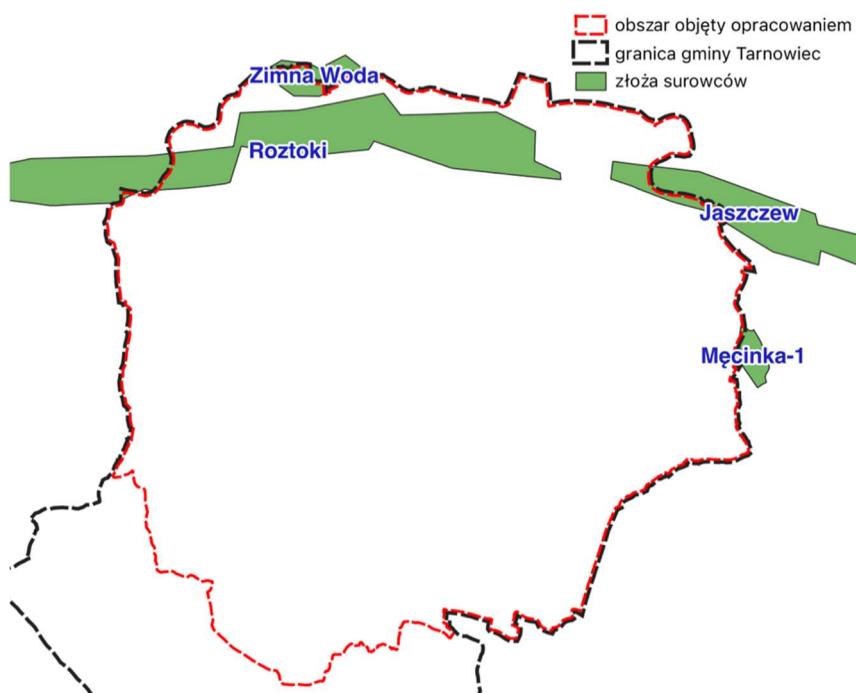
Rysunek 4 Złóża surowców naturalnych na terenie objętym planem
