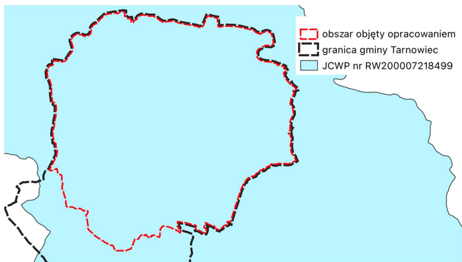
Rysunek 6 Położenie obszaru objętego planem pod względem zlewni Jednolitych Części Wód Powierzchniowych
