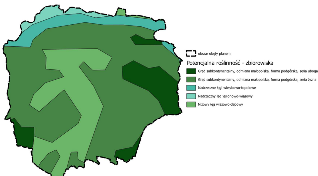
Rysunek 7 Potencjalna roślinność naturalna obszaru objętego planem na podstawie: Matuszkiewicz J.M., Wolski J., 2023, Potencjalna roślinność naturalna Polski (wersja wektorowa), IGiPZ PAN, Warszawa.
