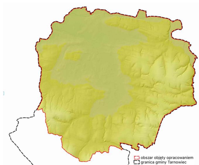
Rysunek 3 Ukształtowanie terenu na obszarze objętym planem
