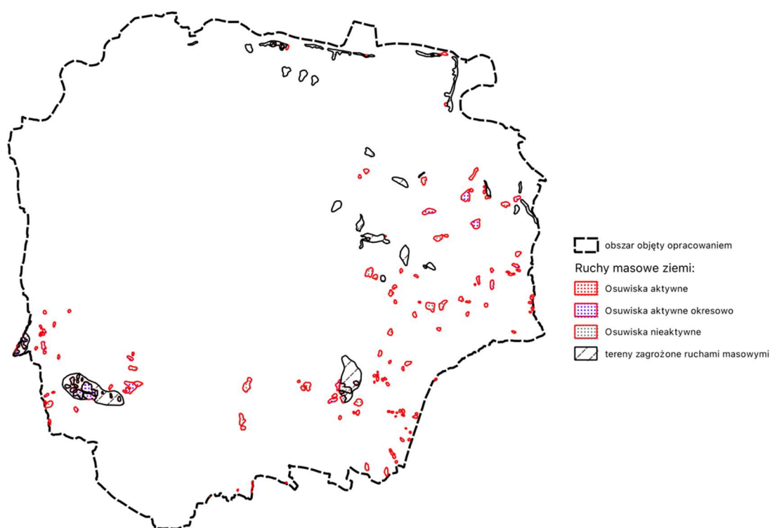
Rysunek 10 Tereny osuwisk aktywnych, aktywnych okresowo i nieaktywnych oraz obszary zagrożone ruchami masowymi na terenie objętym planem (opracowanie własne na podstawie map SOPO)
